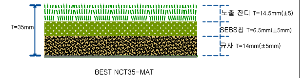
인조잔디 상세도
