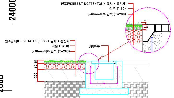
인조잔디 단면도
